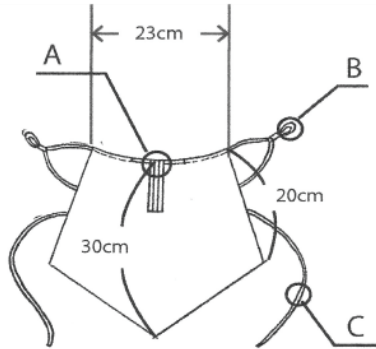
〔図A〕展開図
